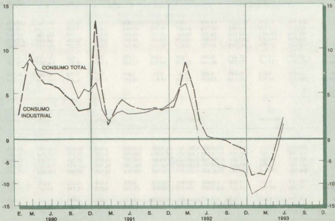
GRAFICO 12 Energía eléctrica: consumo total e industrial en 24 ciudades VARIACIONES PORCENTUALES ANUALES*
