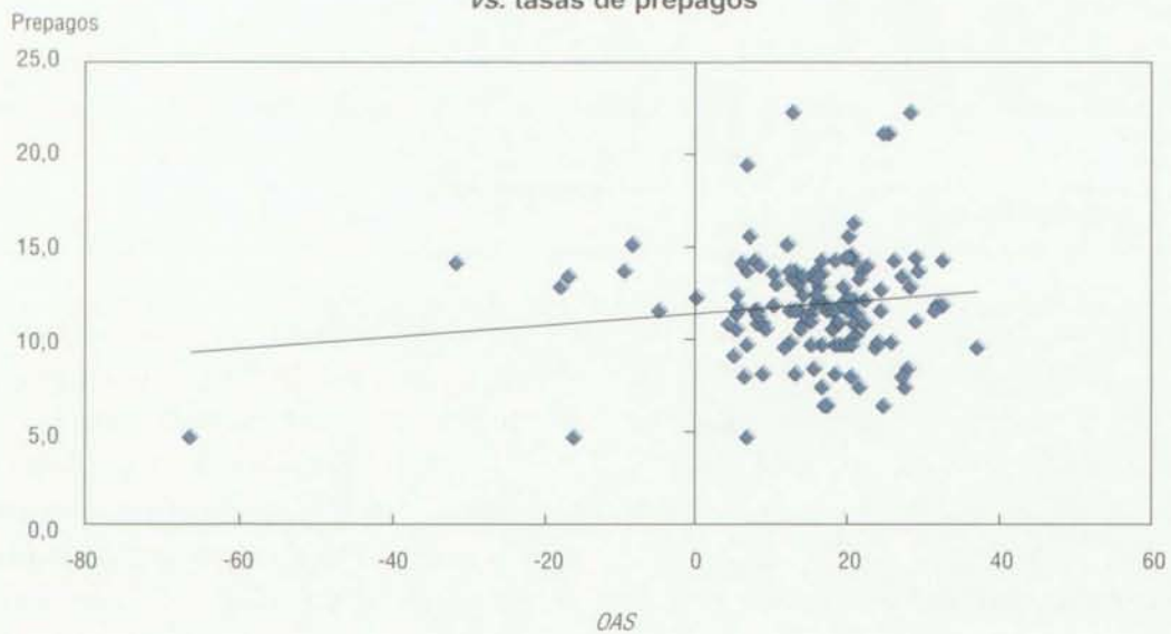
Gráfico 3 OAS en puntos básicos vs. tasas de prepagos
