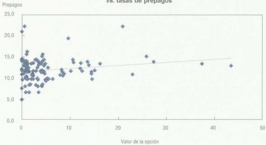
Gráfico 2 Valor de la opción en puntos básicos vs. tasas de prepagos
