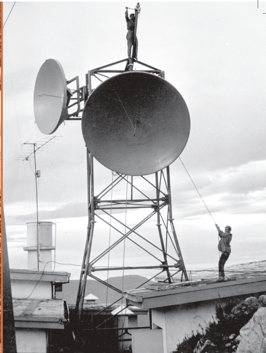
En el municipio de Ábrego (Norte de Santander) se instaló la estación Jurisdicciones que recibía la transmisión del nevado del Ruiz y fue el enlace por bandas de alta frecuencia (VHF) más extenso del mundo (400 km).
